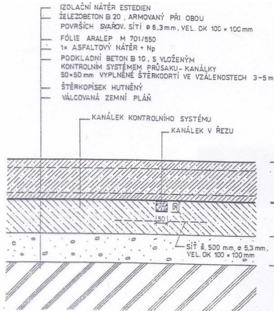
Kontrolní systém – kanálky Skladba s betonovým povrchem
