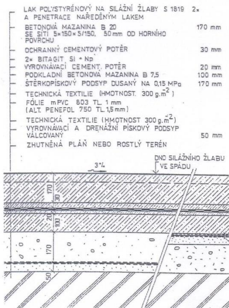
Varianty plošné kontrolní drenáže Skladba s betonovým povrchem
