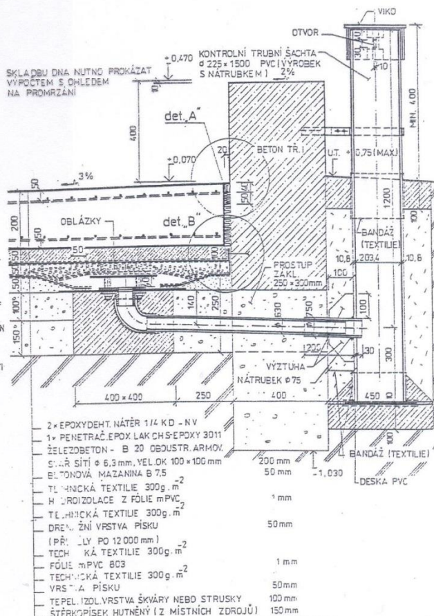
Detail napojení kontrolní šachty
