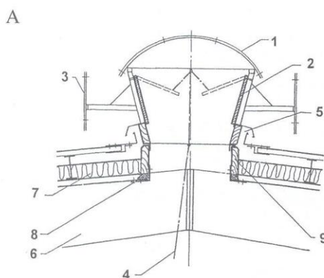
Obrázek 17: Příklad řešení větracího otvoru přirozeného větrání stáji - hřebenová větrací štěrbinu (1 - stříška z transparentního materiálu, 2 - ventilační klapka, 3 - ochranná clona proti větru, 4 - ovládací mechanismus, 5 - odvětrání tepelně izolovaného střešního pláště, 6 - nosný střešní rám, 7 - tepelná izolace na podhledovém plechu, 8 - těsnění mezer PUR pěnou, 9 - krycí fošna)
