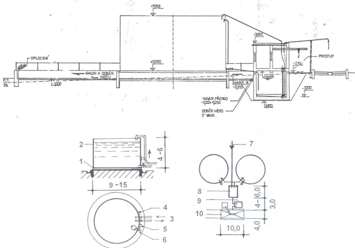
SCHEMA SKLADU KEJDY 2500 m 3 SE ZÁCHYTNOU VANOU SE ZVÝŠENÝMI OBRUBNÍKY
