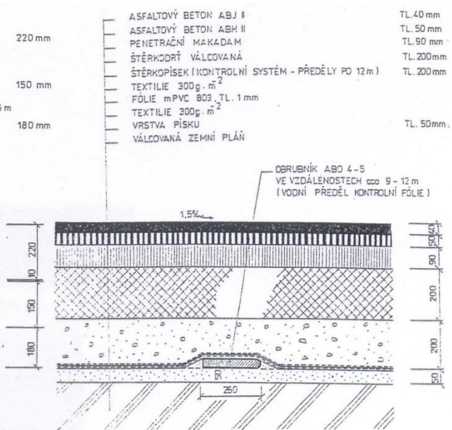
Úprava rozvodí kontrolního systému Skladba s asfaltobetonovým povrchem
