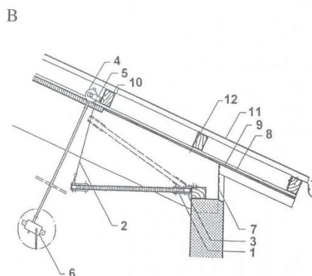
Obrázek 18: Příklad řešení větracího otvoru přirozeného větrání stáji - stěnová štěrbinu pro regulovaný přívod vzduchu (1 - větrací klapka, 2 - popruh, 3 - kloubové uchycení, 4 - naviják popruhu, 5 - třmen, 6 - pohon, 7 - ochranná mřížka, 8 - záklop z prken, 9 - laťování, 10 - krokev, 11 - vláknocementová vlnitá střešní krytina, 12 - nosný střešní rám)
