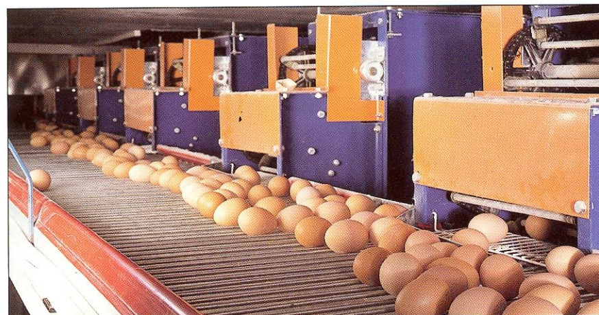
Eiübergabe auf den Quersband
