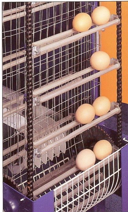
Elevátor – hier geöffnet
